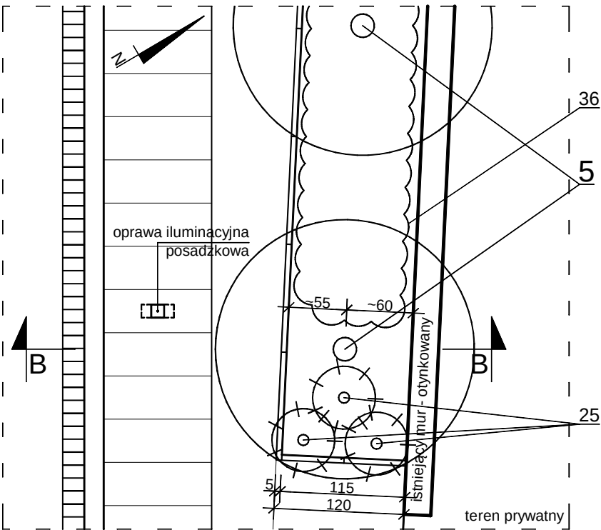
RZUT:
