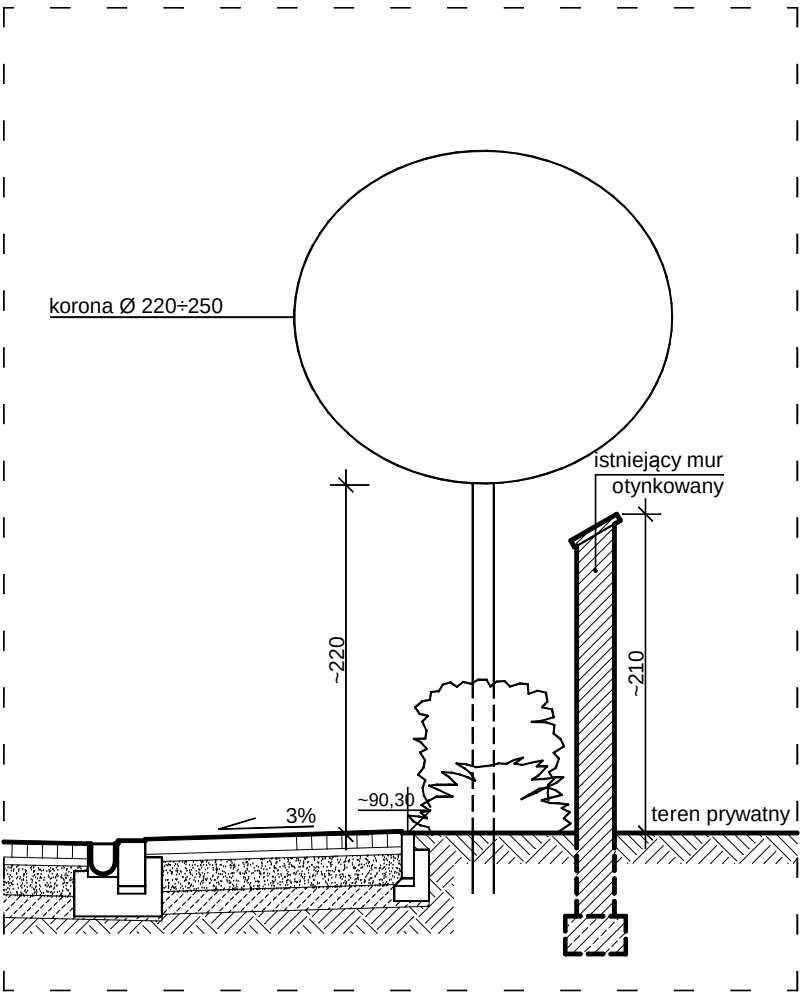
PRZEKRÓJ B-B:
