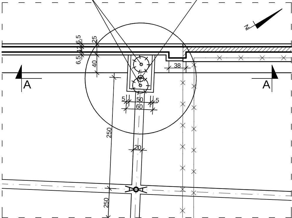
RZUT:
