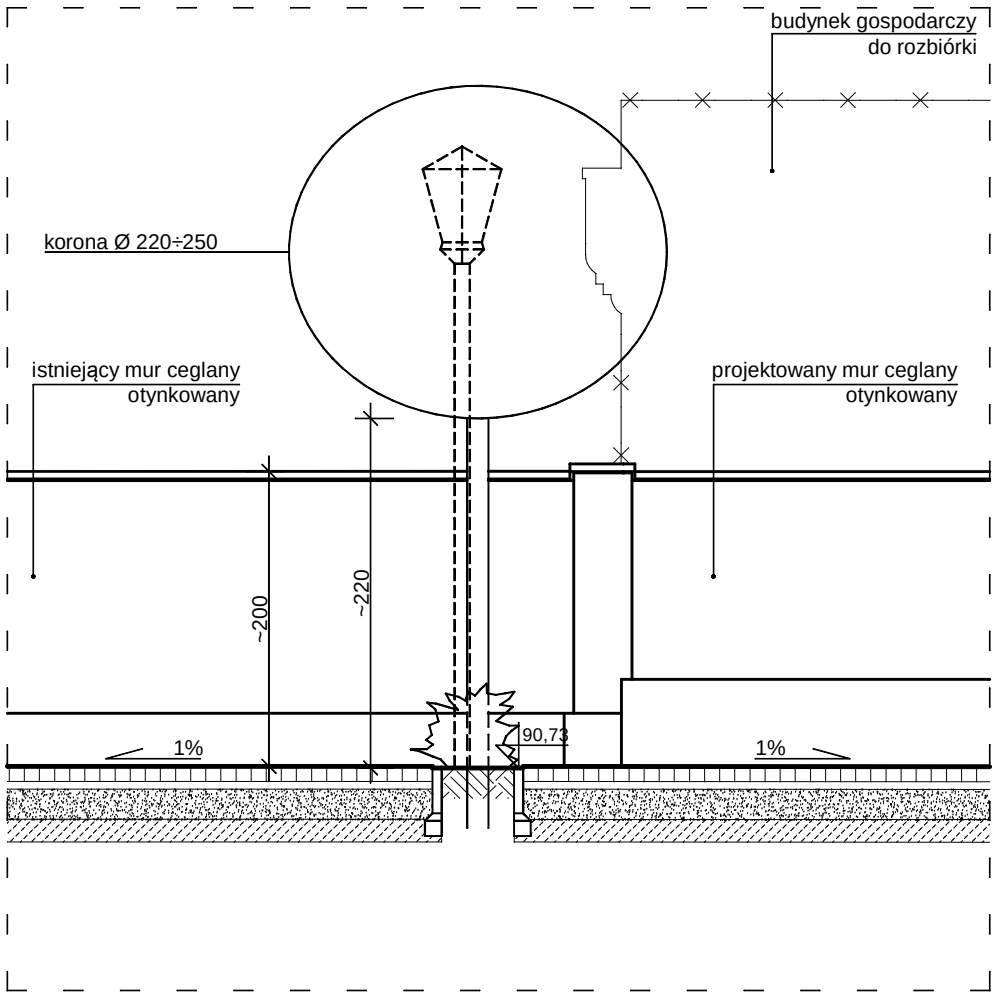
PRZEKRÓJ A-A:
