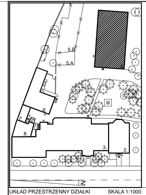
UKŁAD PRZESTRZENNY DZIAŁKI SKALA 1:1000
