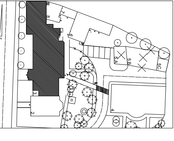
UKŁAD PRZESTRZENNY DZIAŁKI SKALA 1:1000
