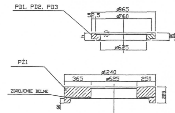
STUDZIENKA KANALIZACYJNA typ TB 1000
