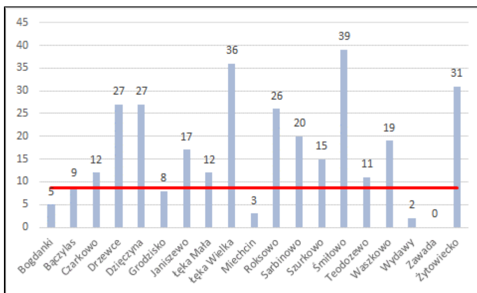
Wykres 4. Podmioty gospodarcze na terenie sołectw Gminy Ponec
