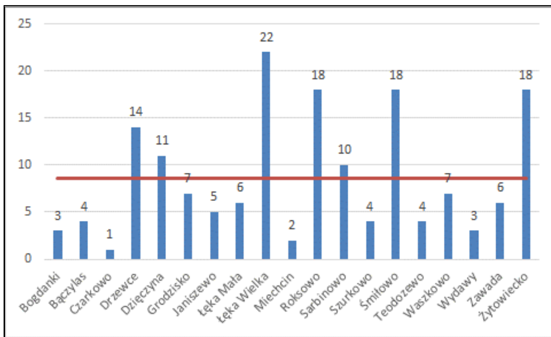
Wykres 3. Liczba osób bezrobotnych na terenie Gminy Poniec
