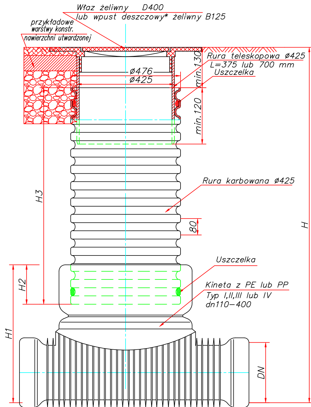
Studzienka inspekcyjna Ø425 z rurą teleskopową i wjazdem żeliwnym lub wpustem klasy B lub D
